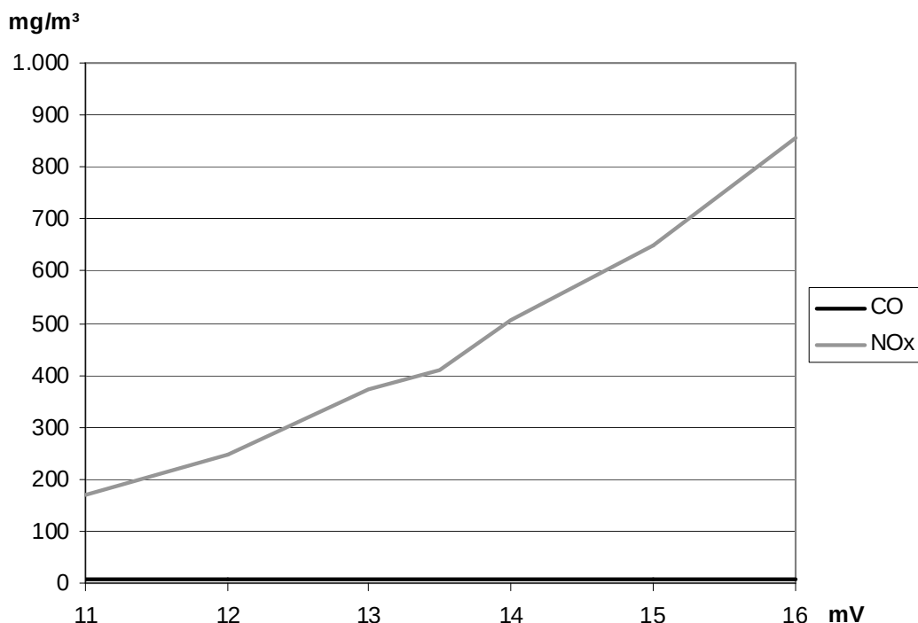
Abbildung 4, Beispielhafter Schadstoffverlauf über Lambdasondenspannung im Magerbetrieb
